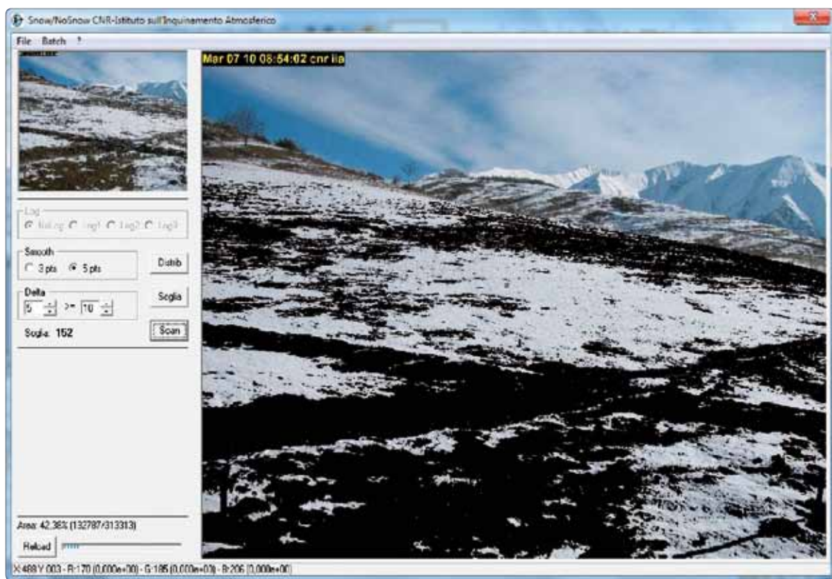
Fig. 4 - Schermata di Snow-noSnow per l'analisi della immagine di Monti della Laga.
