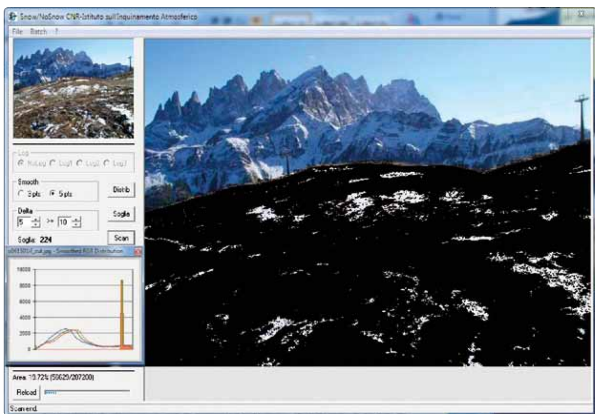
Fig. 5 - Schermata di Snow-noSnow per l'analisi della immagine di Cima Pradazzo.
