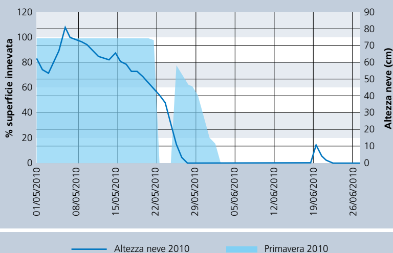
Fig. 11 - Altezza neve misurata a Cima Pradazzo e variazione temporale della estensione della copertura nevosa nell'area indicata in Fig. 07 nella primavera 2009. I picchi a zero della copertura nevosa sono dovuti alla mancanza di foto in data base per problemi di trasmissione delle immagini via GSM.
