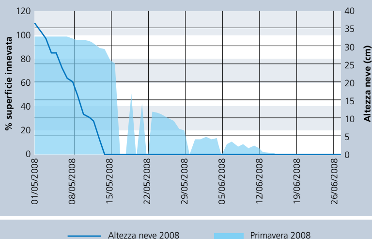
Fig. 10 - Altezza neve misurata a Cima Pradazzo e variazione temporale della estensione della copertura nevosa nell'area indicata in Fig. 07 nella primavera 2008. I picchi a zero della copertura nevosa sono dovuti alla mancanza di foto in data base per problemi di trasmissione delle immagini via GSM.
