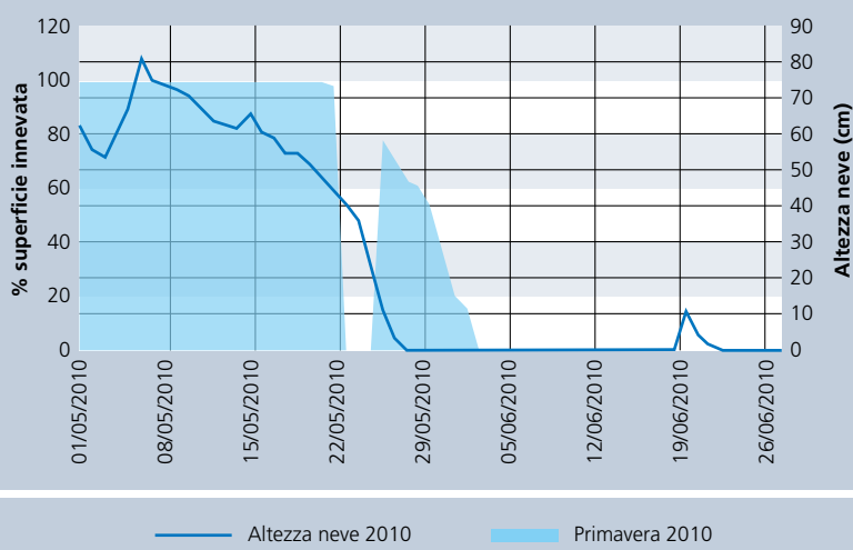
Fig. 12 - Altezza neve misurata a Cima Pradazzo ed variazione temporale della estensione della copertura nevosa nell'area indicata in Fig. 07 nella primavera 2010. I picchi a zero della copertura nevosa sono dovuti alla mancanza di foto in data base per problemi di trasmissione delle immagini via GSM.
